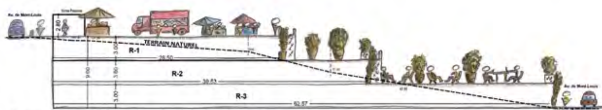
Coupe Longitudinale de Principe
