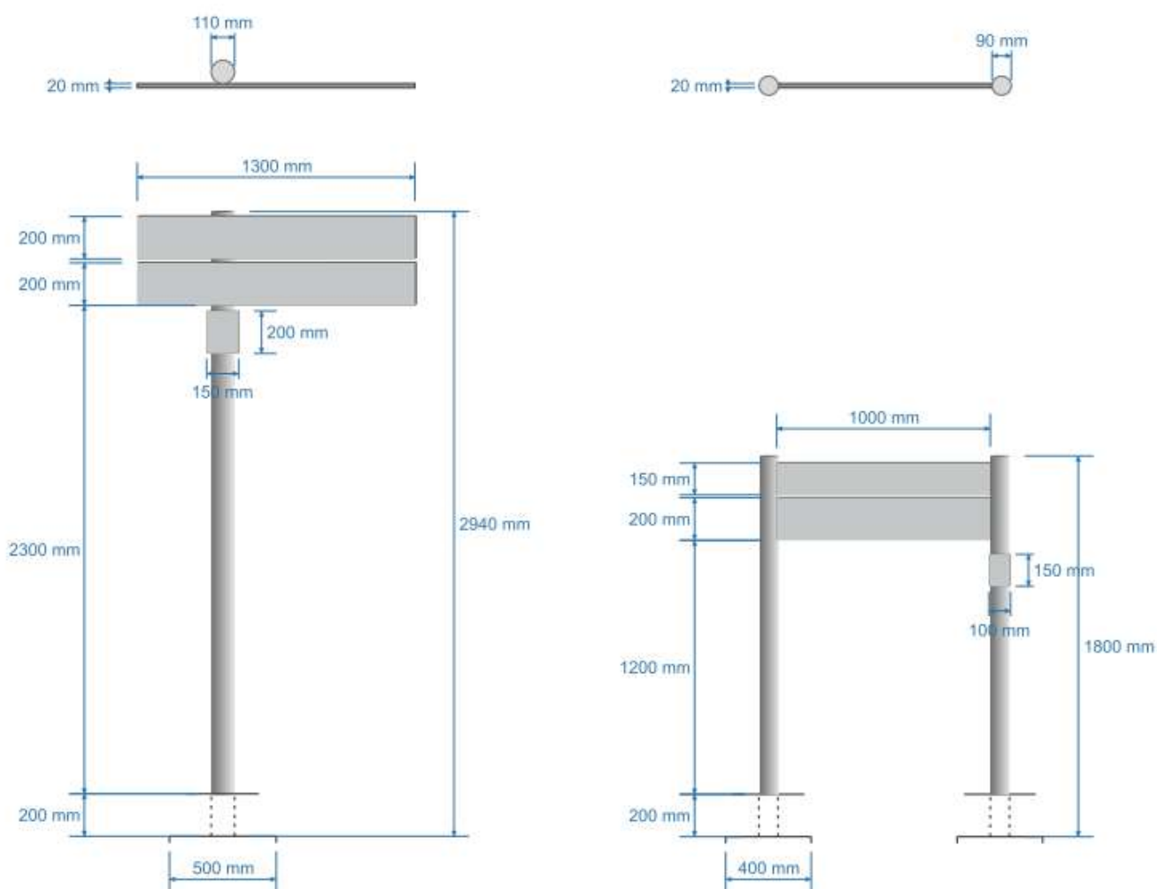
Dimensions des matériels en ALUMINIUM
